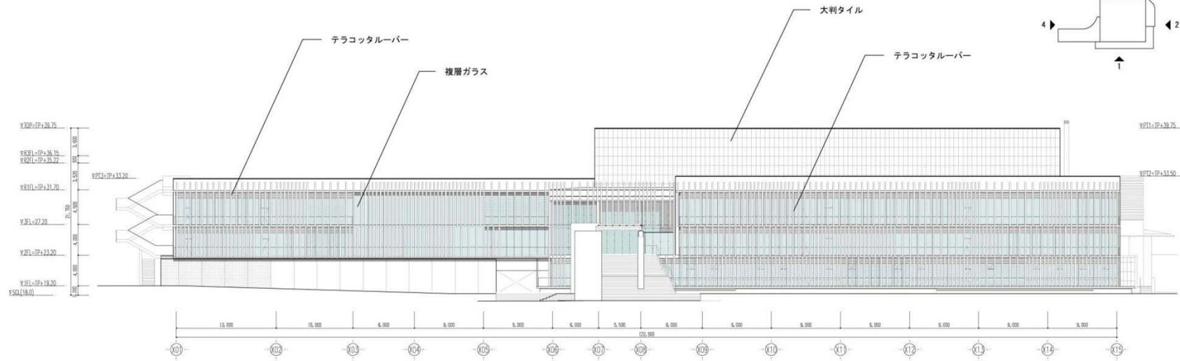
1 北西立面図
