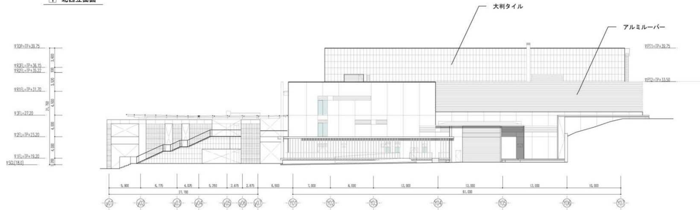
1 北西立面図
